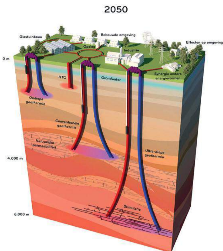
Schematische weergave van het winnen van aardwarmte.
